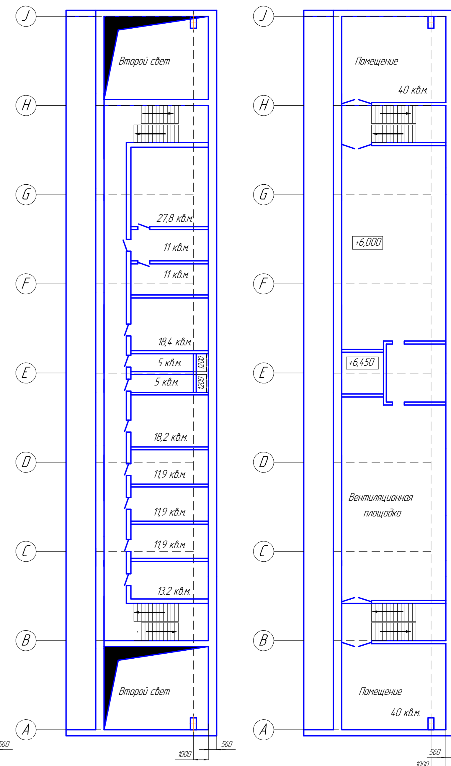
План 2 этажа на отм. ± 3.000
