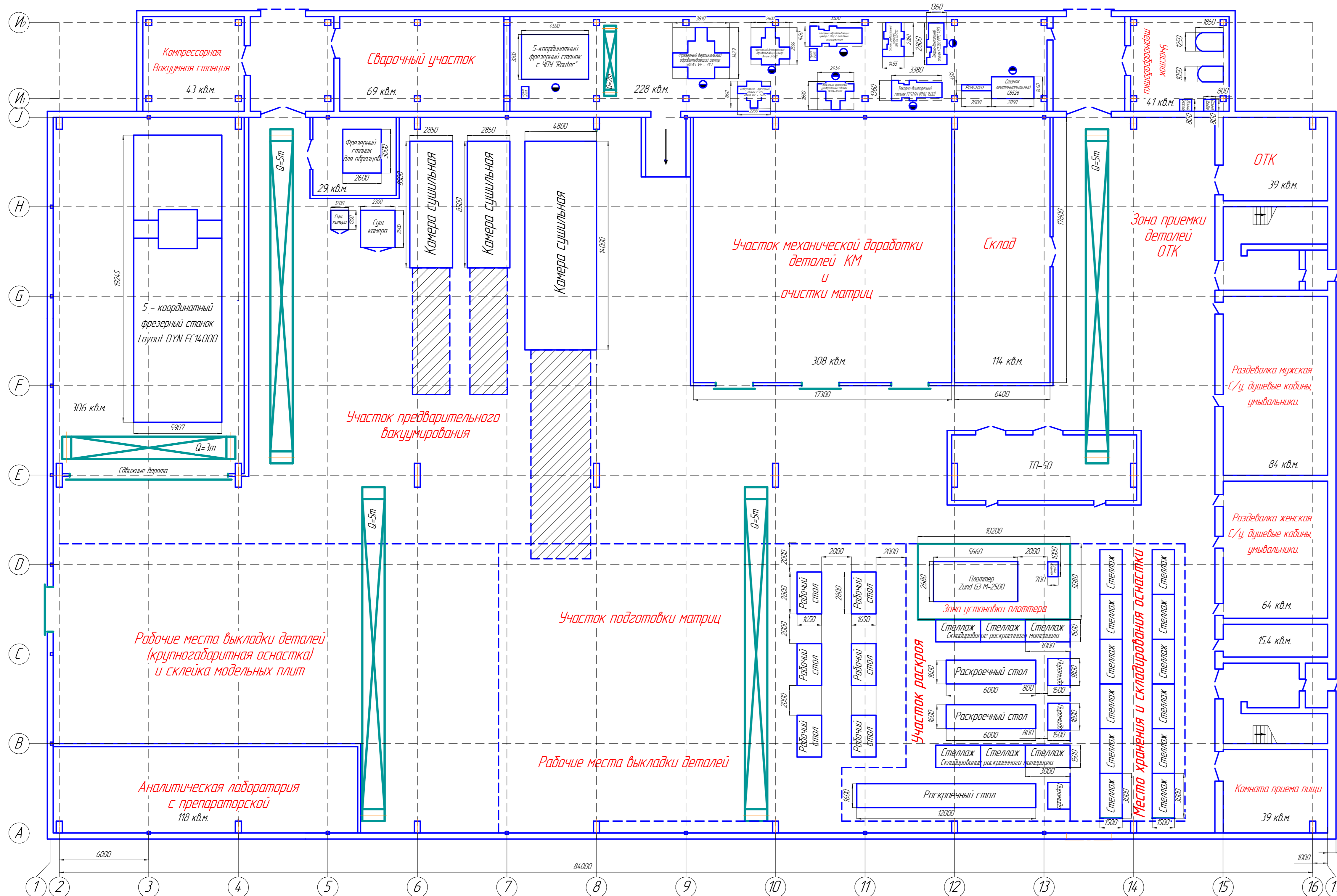
План 1 этажа на отм. ± 0.000
